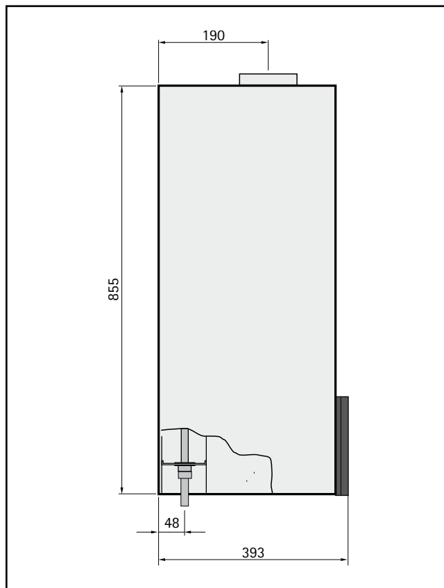
rozmery prípojok
