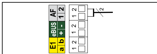
pripojenie vonkajšieho snímača
