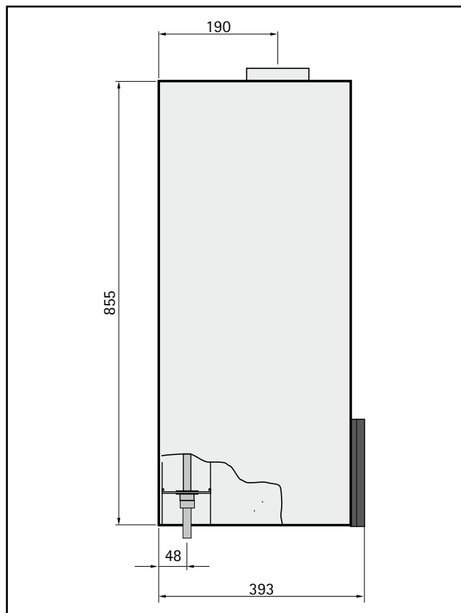
rozмеры присоединения
