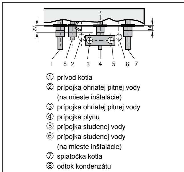
prípojky kotla
