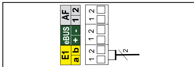
pripojenie priestorového termostatu – beznapät'ové pripojenie
