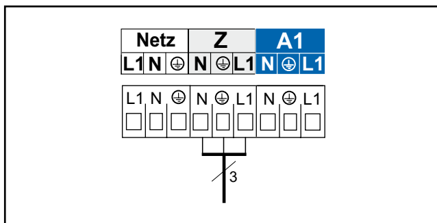
pripojka obehového čerpadla (externé príslušenstvo)
