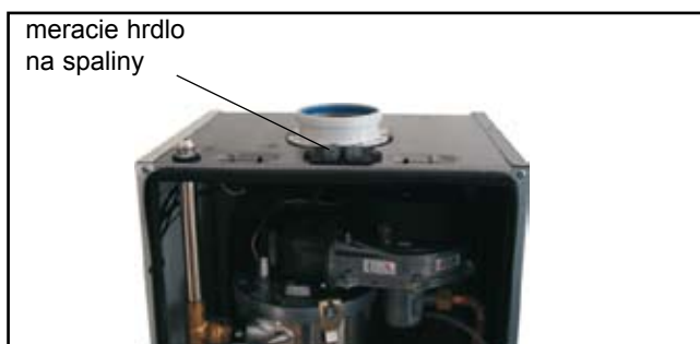
meranie spalín na kotle bez plášťa
