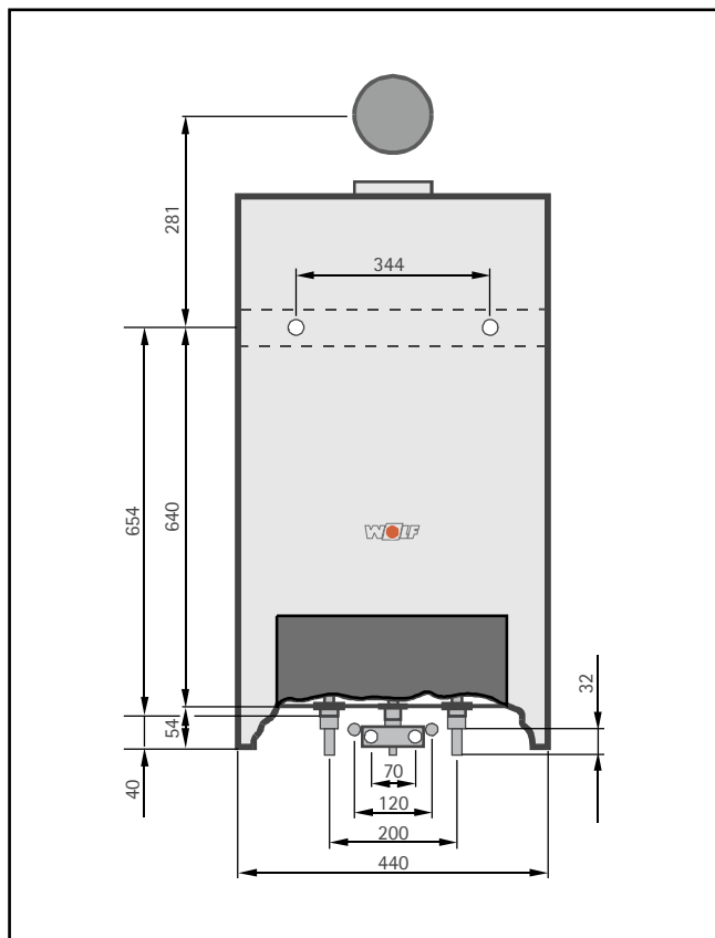
rozmery prípojok
