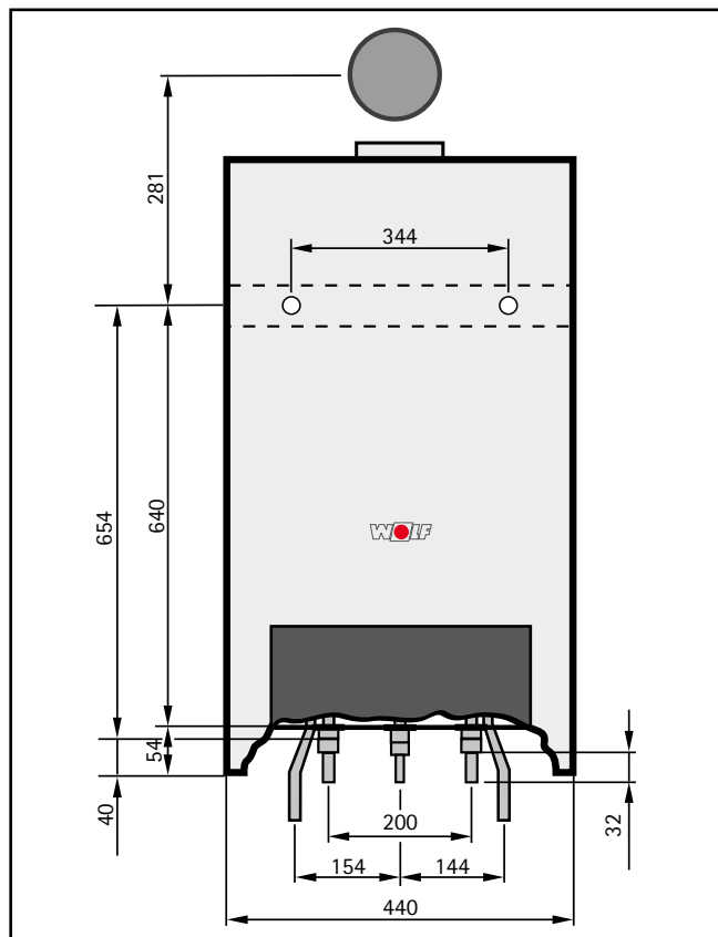
rozмеры присоединения
