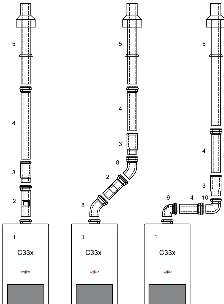
Príklady na pripojenie nezávislé od vzduchu v miestnosti (zvislé)
