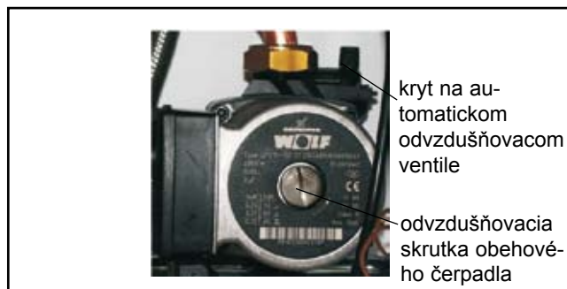
automatický odvzdušňovací ventil na obehovom čerpadle
