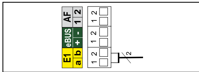
pripojenie priestorového termostatu
