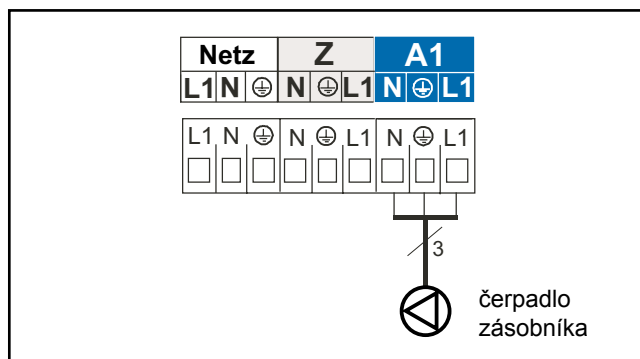
pripojenie výstupu A1
