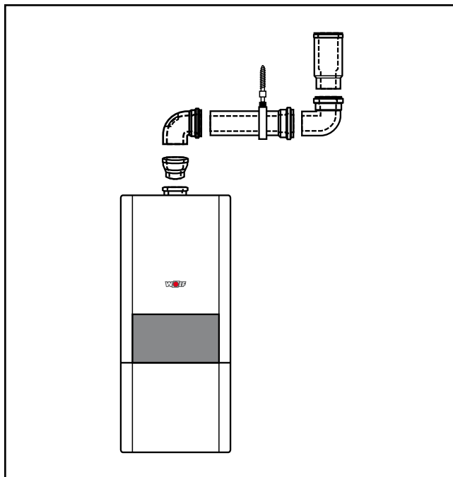
príklad združeného vedenia spaliny / vzduch
