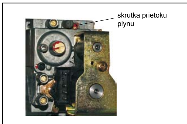
plynový kombiventil
