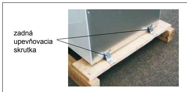
upevnenie na palete zozadu
