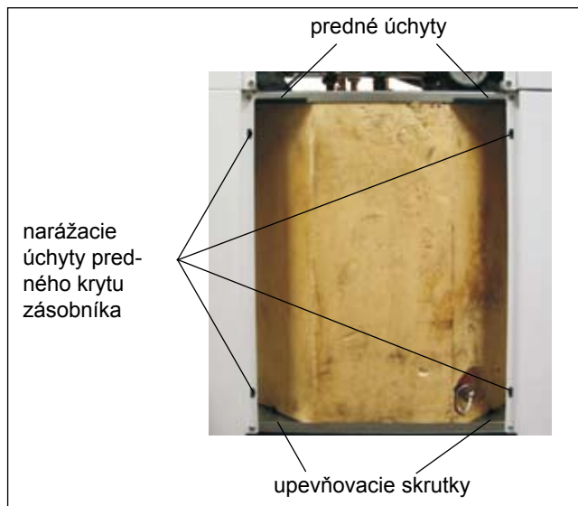
odkrytý zásobník spredu
