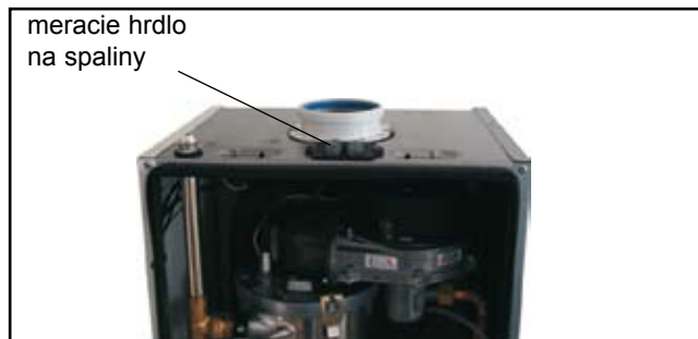
meranie spalín na kotli bez plášťa
