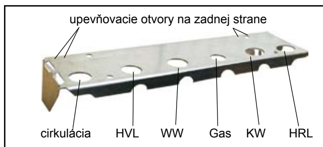
konzola s ohnutými bočnicami nadomietková montáž (príslušenstvo)
