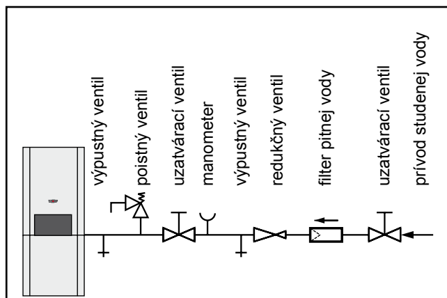
odporúčané riešenie prívodu studenej vody
