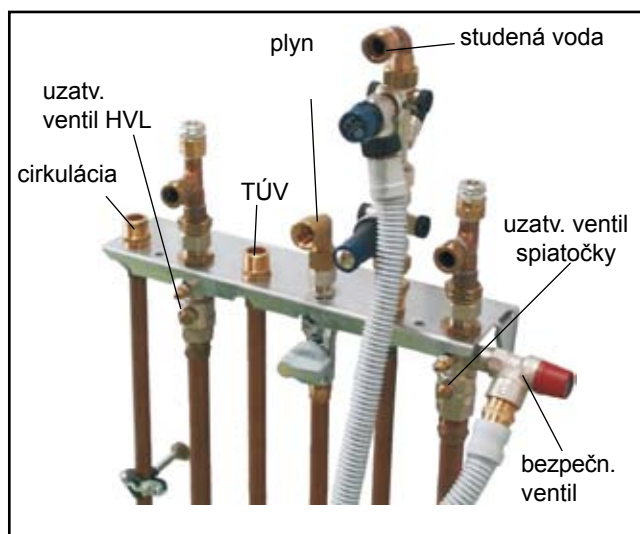
ventily na konzole nadomietková montáž (príslušenstvo)
