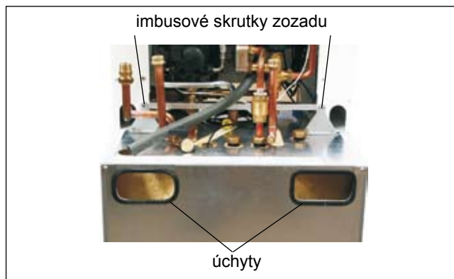
upevnenie na palete zozadu
