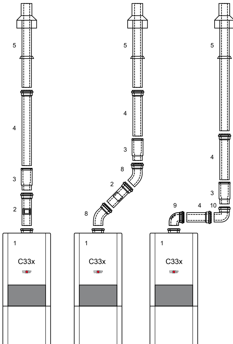
Príklady na pripojenie nezávislé od vzduchu v miestnosti (zvislé)
