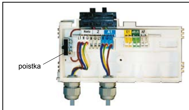
skrinka regulácie vyklopená, otvorený kryt svorkovnice
