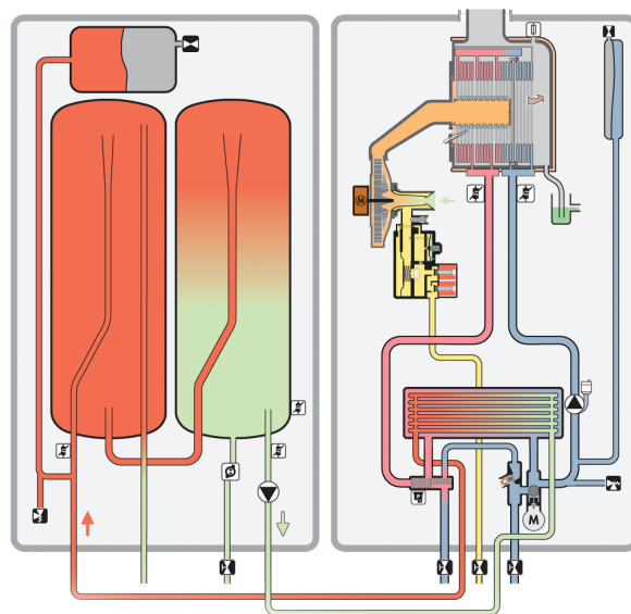
Nahrievanie zásobníka v zostave VUI bez odbere teplej vody
