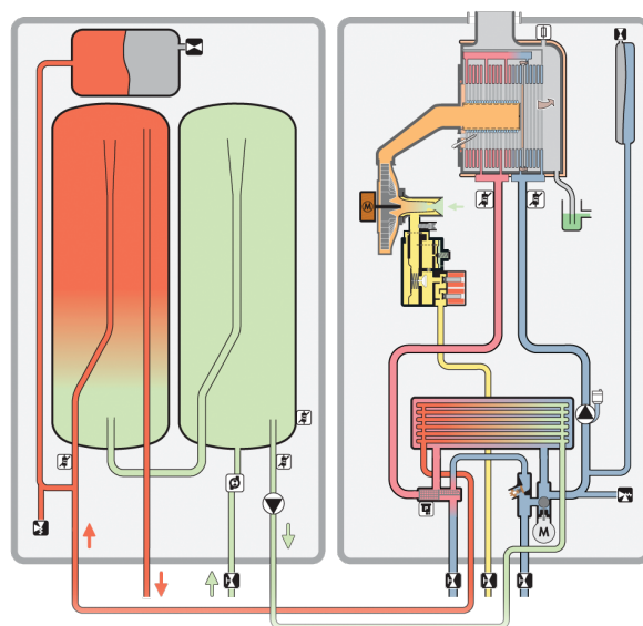
Nahrievanie zásobníka v zostave VUI pri súčasnom odbere teplej vody
