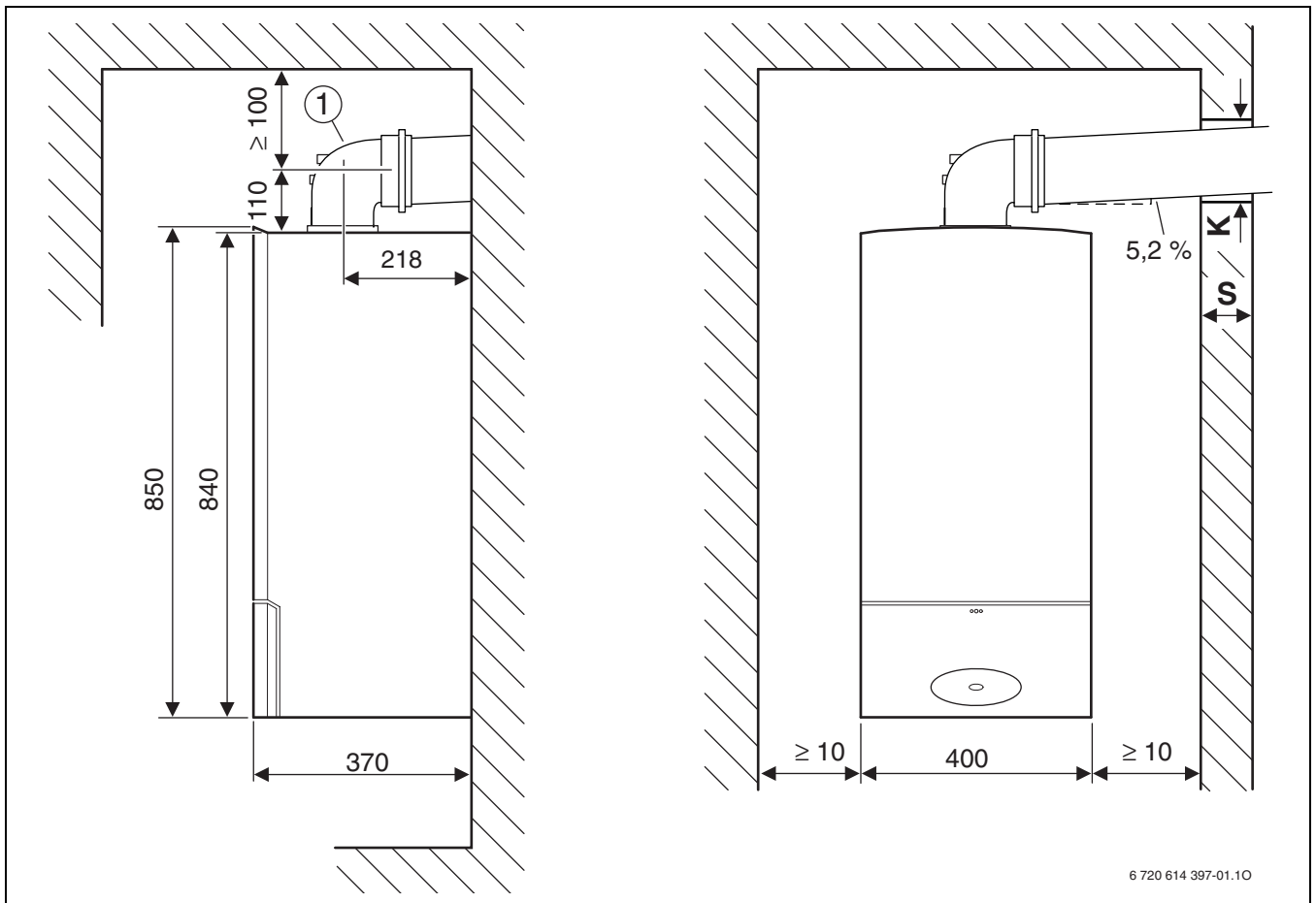
Obr. 5 Vedenie odvodu spalín Ø 80/125 mm alebo Ø 80 mm
