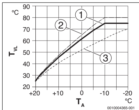
Obr. 20 Nastavenie vykurovacej krivky pre vykurovacie telesá Stúpanie pomocou dimenzačnej teploty T_{AL} a minimálnej vonkajšej teploty T_{A,min}
