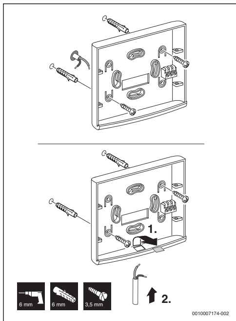
Obr. 9 Inštalácia podstavca
