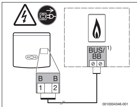
Obr. 10 Pripojenie rádiového modulu ku kotlu
