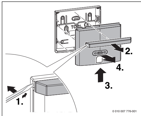
Obr. 8 Sňatie kryty z podstavca
