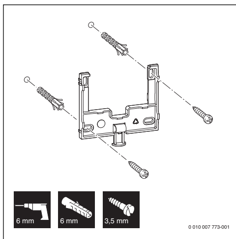
Obr. 13 Inštalácia podstavca
