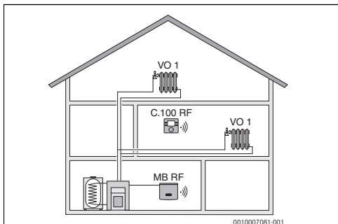
Obr. 1 Příklad vykurovacieho zariadenia s vykurovacím okruhom VO 1 a C 100 RF používanou ako regulátor (v rodinnom dome)
