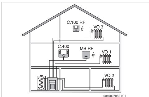
Obr. 2 Příklad vykurovacieho zariadenia s tromi vykurovacími okruhmi a CR 100 RF používanou ako diaľkové ovládanie (rodinný dom s nájomným bytom alebo dielňou)
