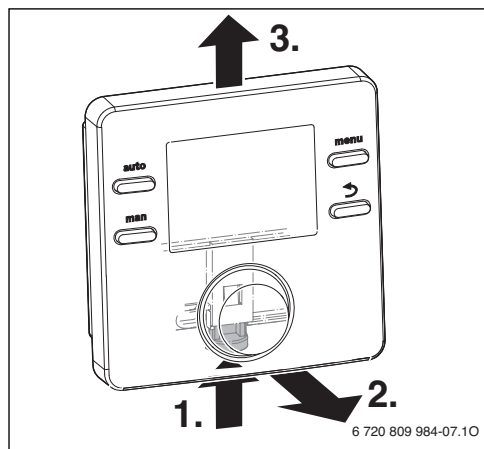
Obr. 15 Demontáž ovládacej jednotky
