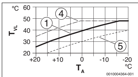
Obr. 19 Nastavenie vykurovacej krivky pre podlahové vykurovanie Paralelný posun prostredníctvom želanej priestorovej teploty
