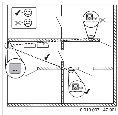
Obr. 12 Miesto inštalácie C 100 RF a rádiového modulu
