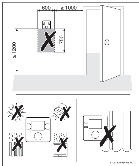
Obr. 11 Miesto inštalácie v referenčnej miestnosti
