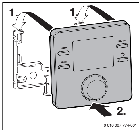
Obr. 14 Zavesenie ovládacej jednotky
