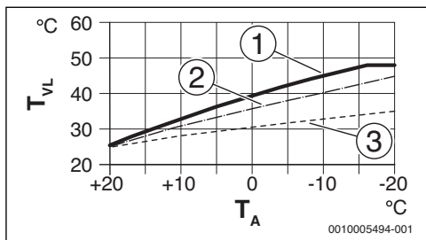
Obr. 18 Nastavenie vykurovacej krivky podlahového vykurovania Stúpanie pomocou dimenzačnej teploty T_{AL} a minimálnej vonkajšej teploty T_{A,min}
