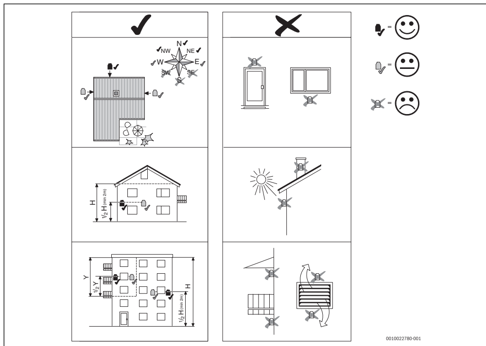
Obr. 16 Miesto inštalácie snímača vonkajšej teploty (severná pologuľa)
