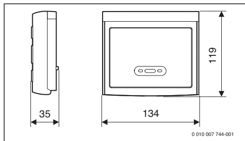
Obr. 6 Bezdrôtový modul MBRF, rozmery v mm
