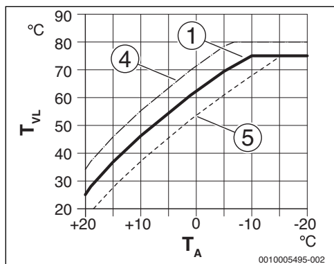
Obr. 21 Nastavenie vykurovacej krivky vykurovacích telies Paralelný posun prostredníctvom želanjej priestorovej teploty
