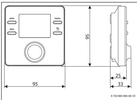
Obr. 5 Ovládací jednotka C 100 RF, rozmery v mm
