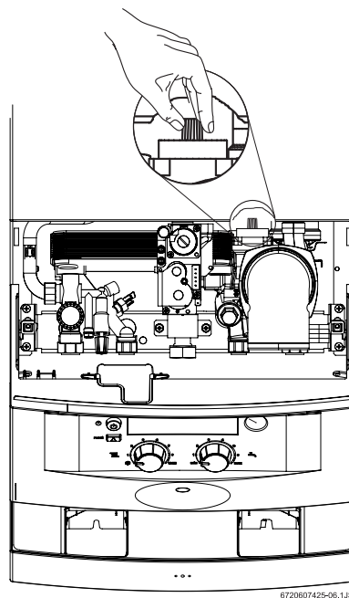
Obr. 15 Odvzdušňovací ventil
