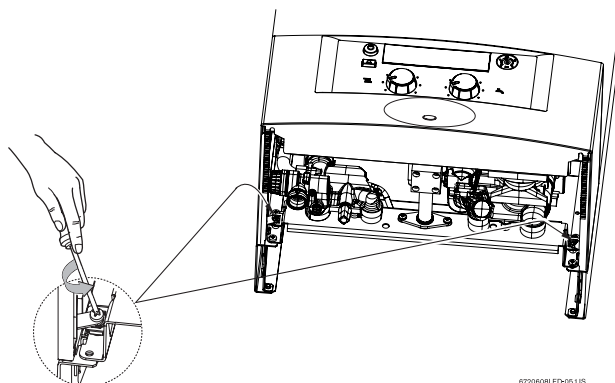
Obr. 8 Zaistovacie skrutky
