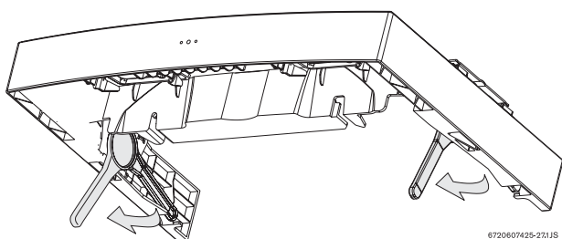
Obr. 12 Upevňovacie páky
