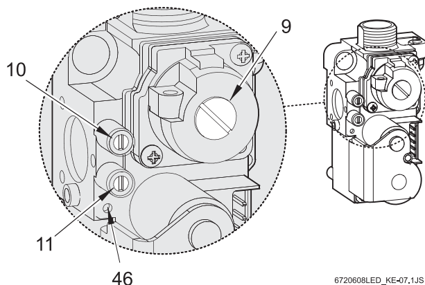
Obr. 28 Plynový ventil
