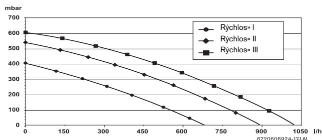
Obr. 5 Charakteristika čerpadla
