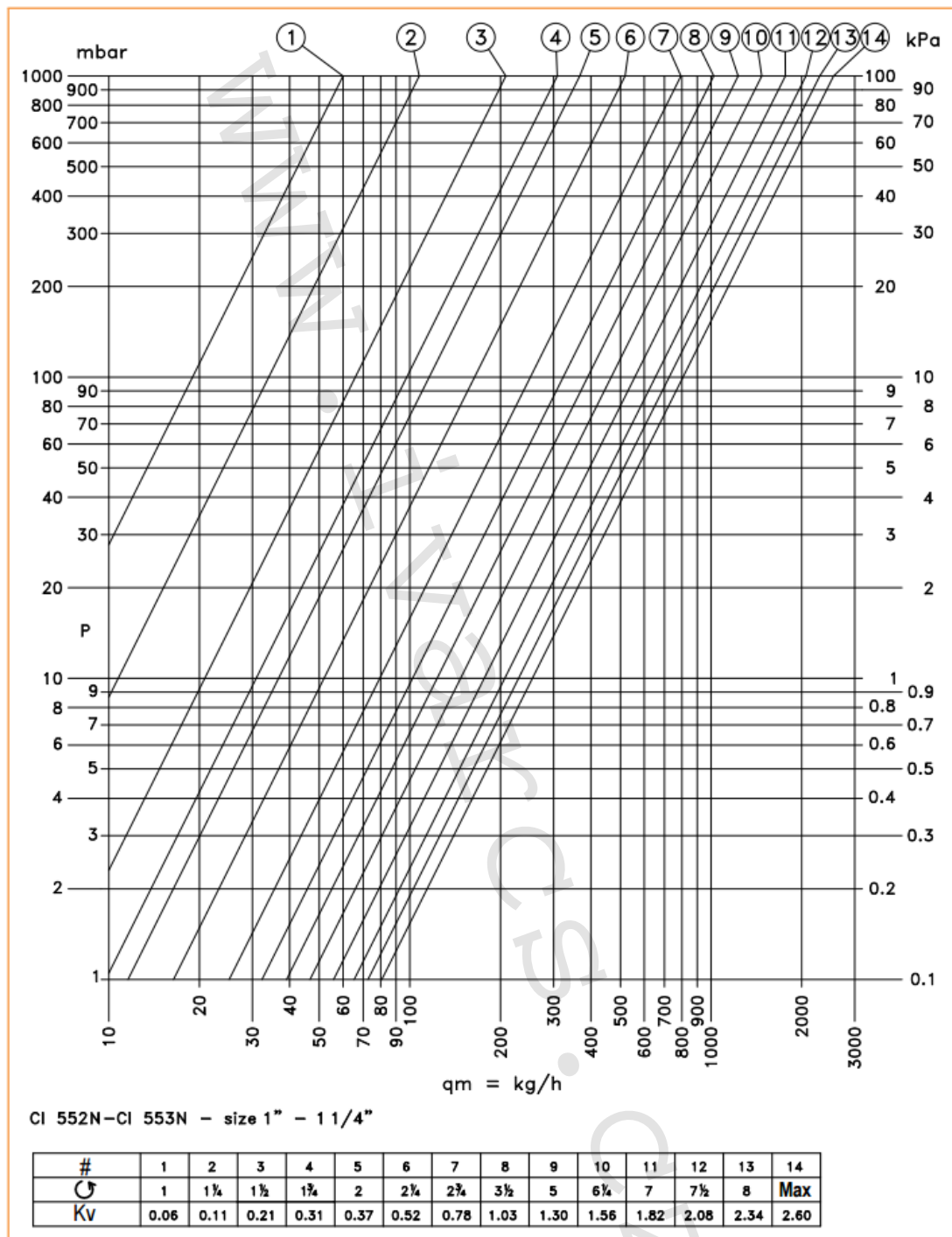
Tabulka nastavitelných hodnot jmenovitého průtoku Kv regulačním šroubením v těle rozdělovače:
