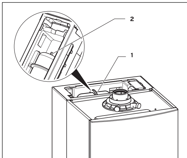
Obr. 8.2 Kontrola plnicího tlaku expanzní nádoby zásobníku
