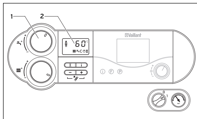
Obr. 7.2 Ukazatel na displeji během ohřevu zásobníku
