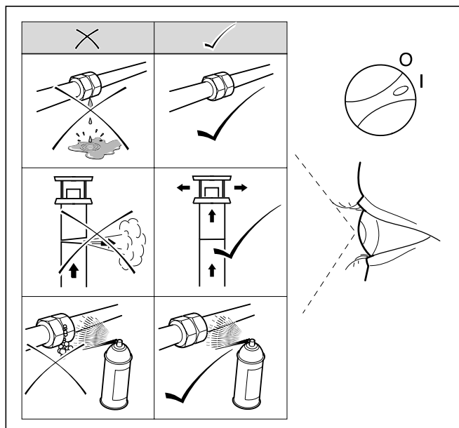
Obr. 8.3 Kontrola funkce
