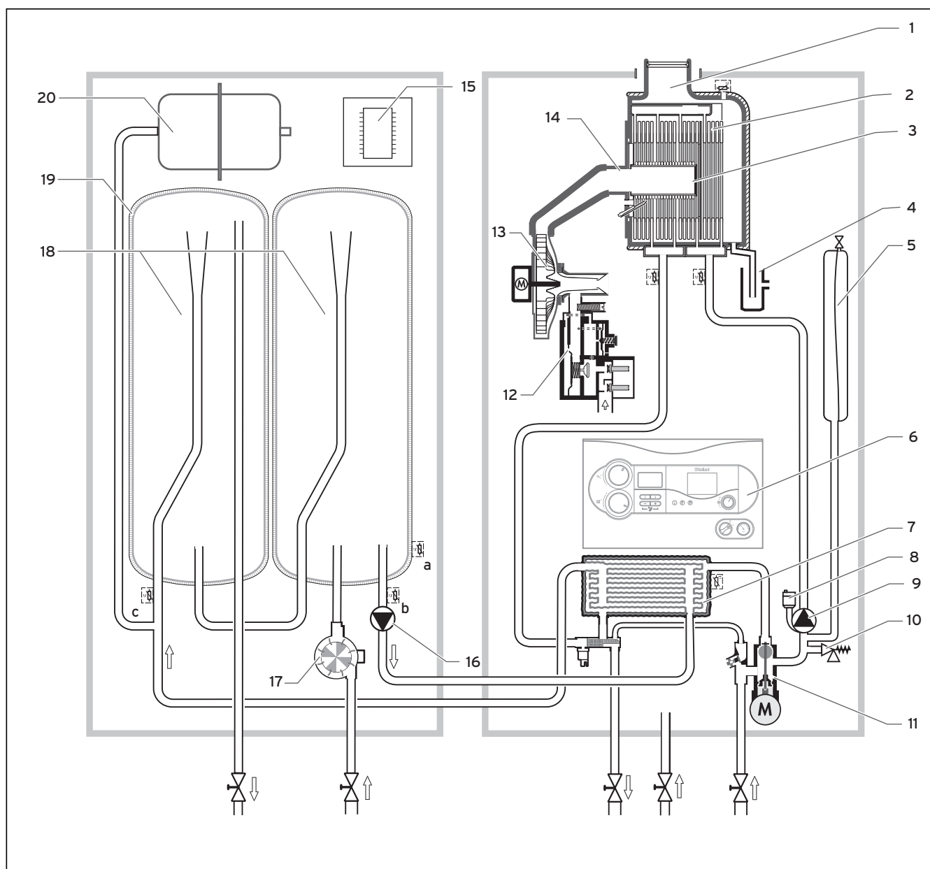
Obr. 2.2 Schéma zařízení
