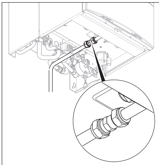
Obr. 5.1 Plynová přípojka
